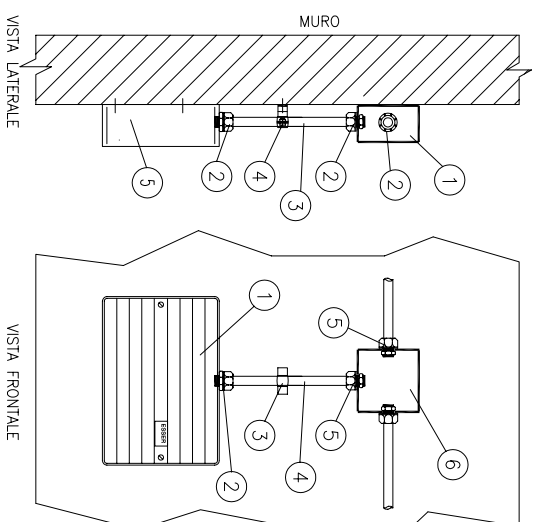
BOX PER TRANSPONDER CON IMPIANTO A VISTA
