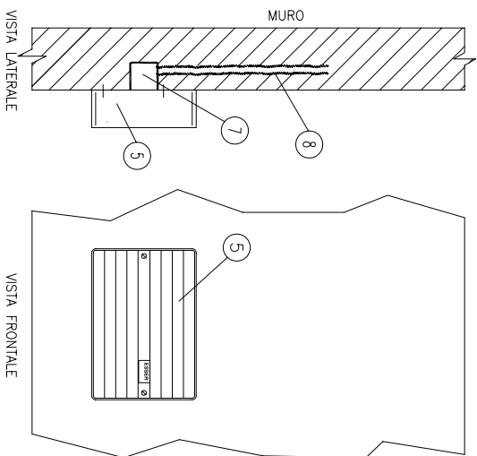
BOX PER TRANSPONDER CON IMPIANTO SOTTO TRACCIA
