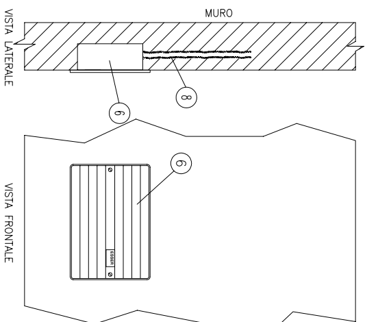
BOX PER TRANSPONDER CON IMPIANTO SOTTO TRACCIA
